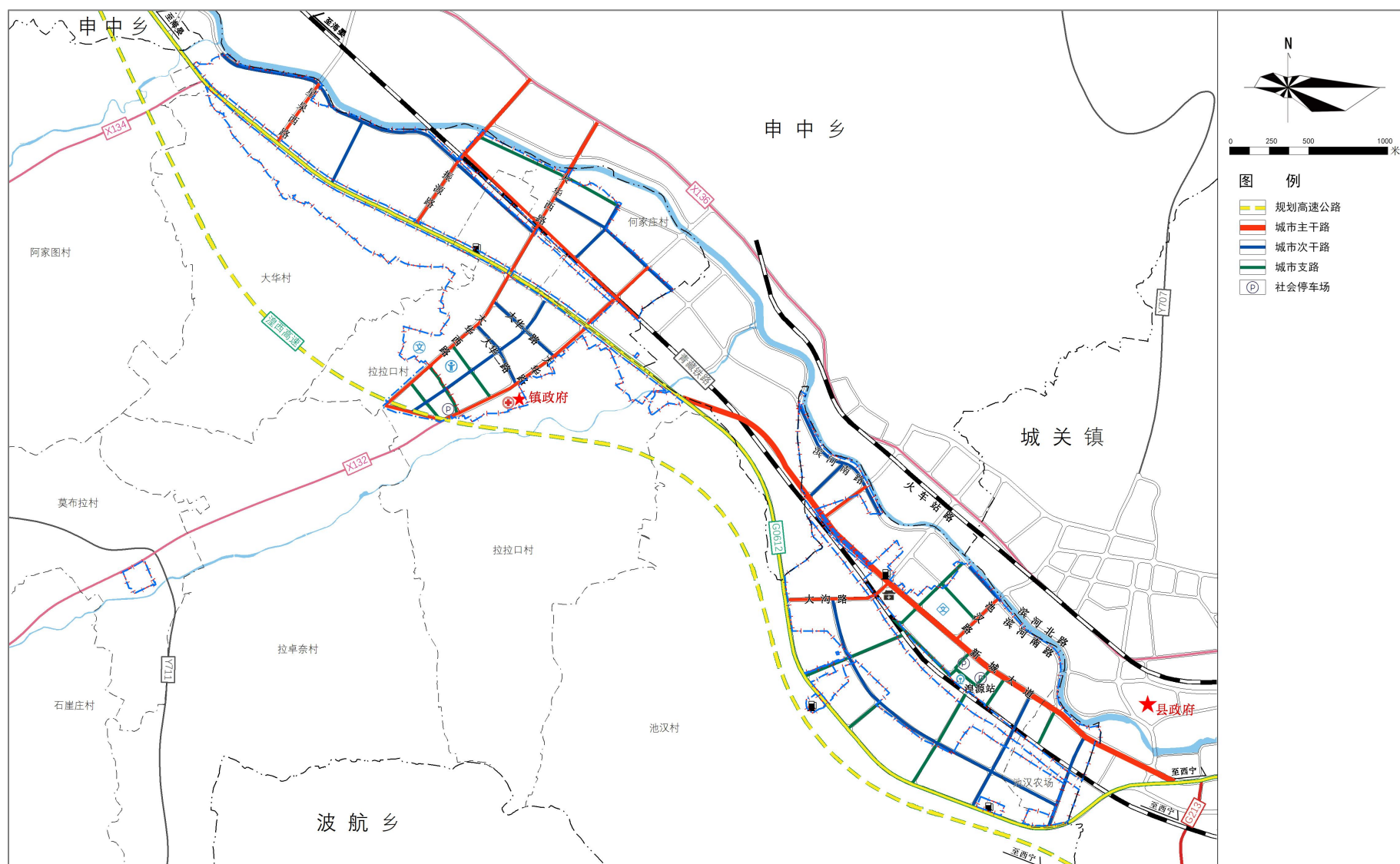
镇政府驻地道路交通规划图
